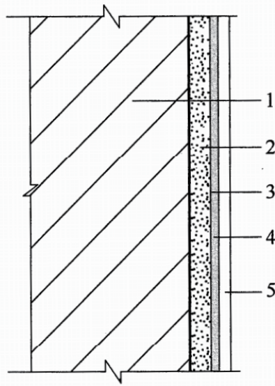
内墙保温采用气凝胶绝热厚型涂料系统时的基本构造 1-墙体基层; 2-腻子层; 3-底涂层; 4-中涂层; 5-面涂层
